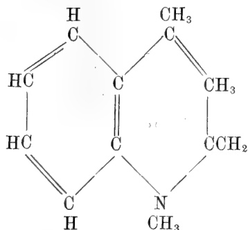
Trimetildiidrochinolina.
